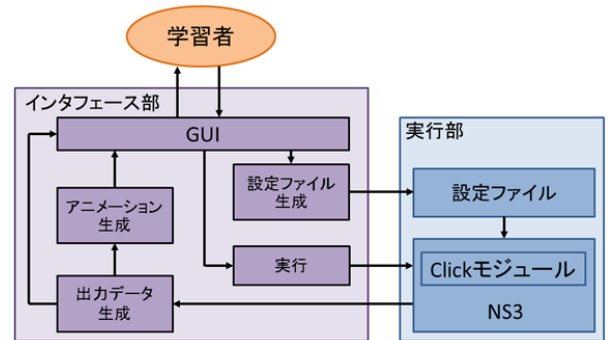
図1 ネットワーク学習システムの概要
