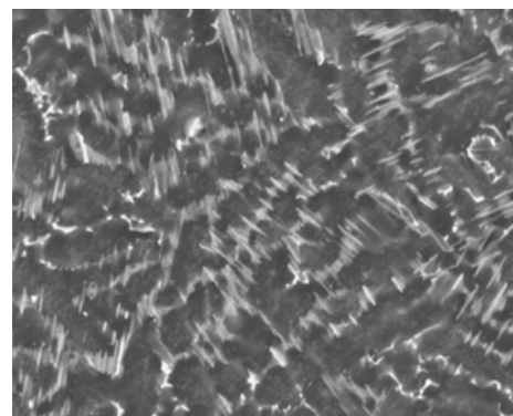
図 1 Mg_{97}Zn_{0.5}Al_{0.5}Gd_2 鑄造合金のラメラ組織。ラメラ組織内に LPSO 相が確認されている。
