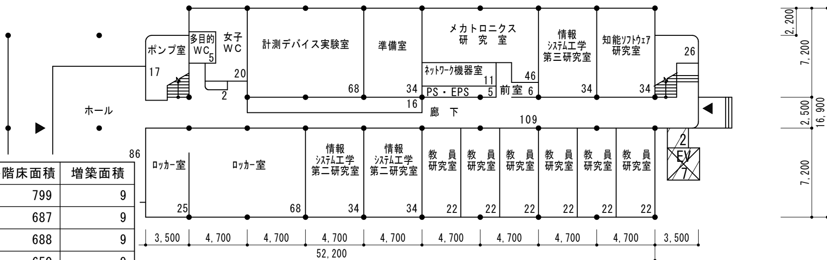
8号棟1階平面図（改修後）S=1/300
