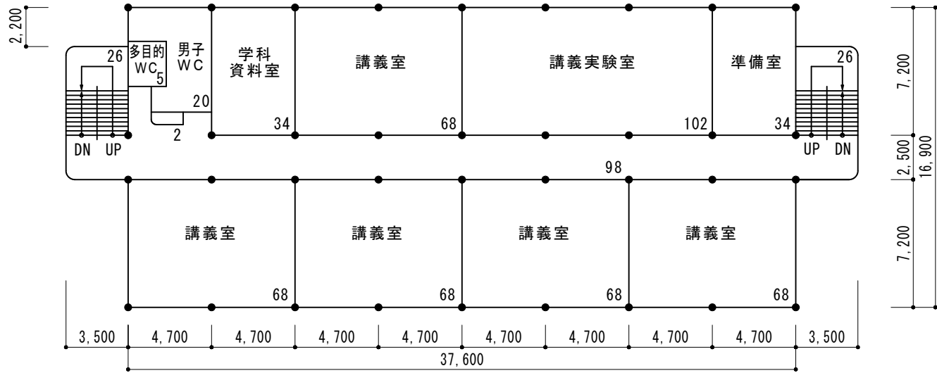
8号棟2階平面図（改修前）S=1/300
