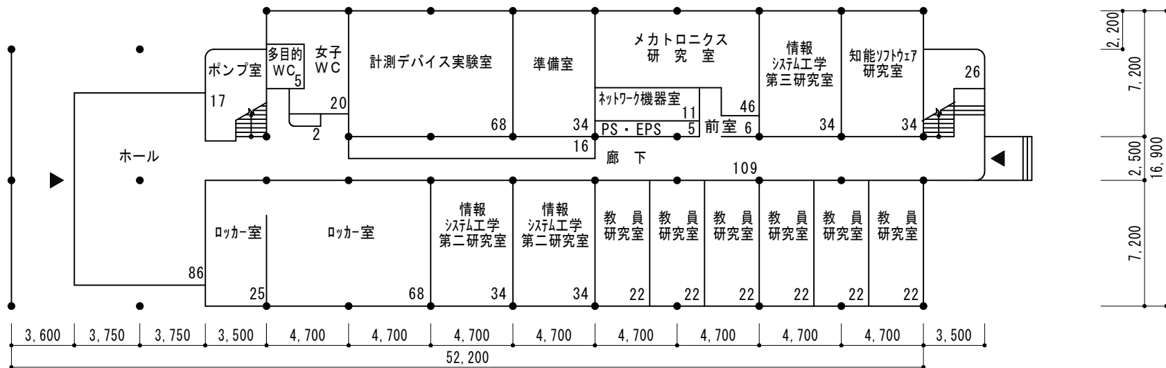
8号棟1階平面図（改修前）S=1/300
