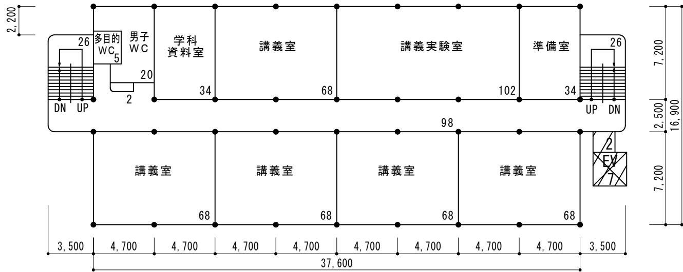
8号棟2階平面図（改修後）S=1/300
