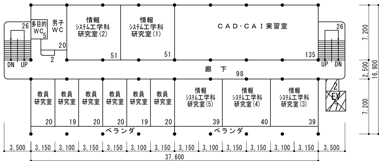
8号棟4階平面図（改修後） S=1/300
