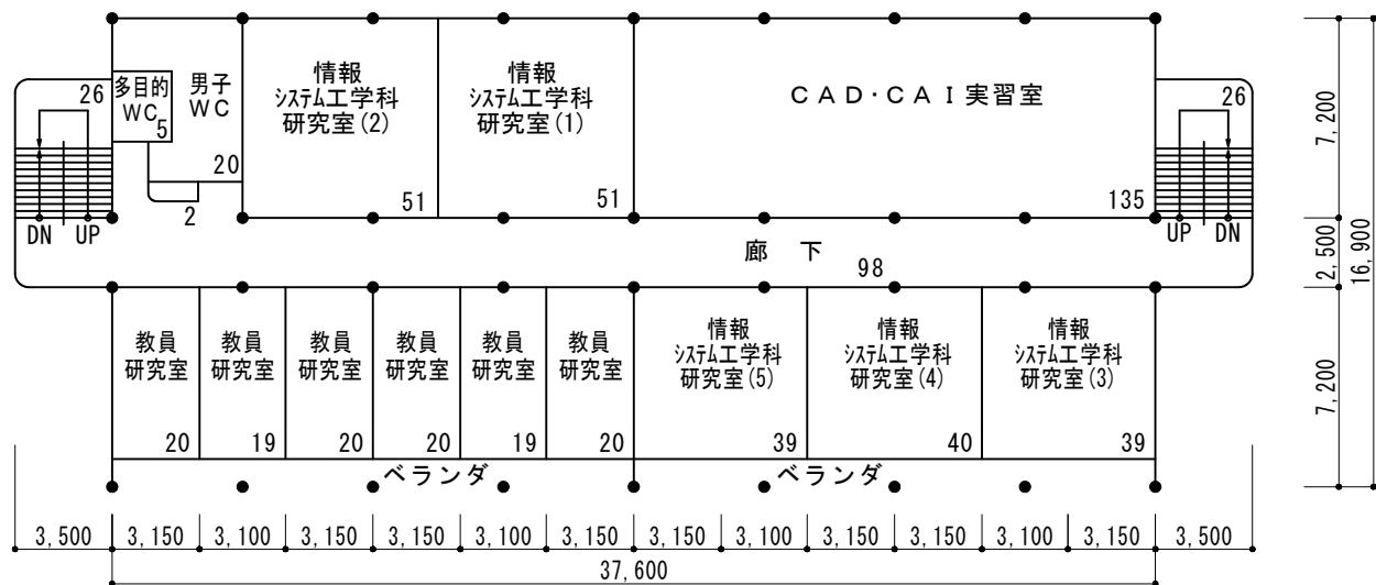
8号棟4階平面図（改修前） S=1/300
