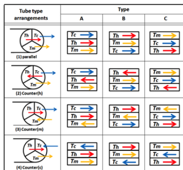
図1 多流体熱交換器の概念
