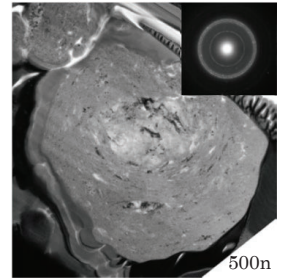
図1 コンバージミル処理したβ型鉄シリサイド粉末の断面組織写真
