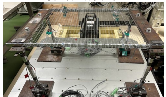
構造物の振動実験
