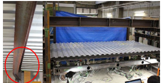
横座屈の再現実験
