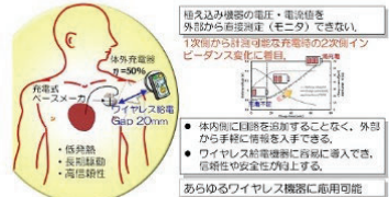
図1 充電状況推定システムの概要
