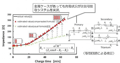
図2 充電状況推定システムの検証
