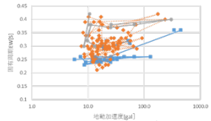
図 3 固有周期と最大加速度の関係
