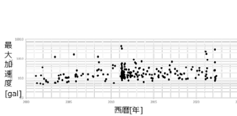
図 1 5 号棟で観測された地震動の最大加速度
