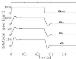
(b) センサベース制御あり
