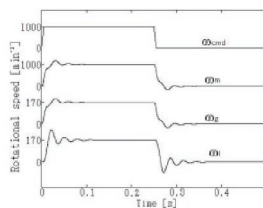
(a) センサベース制御なし
