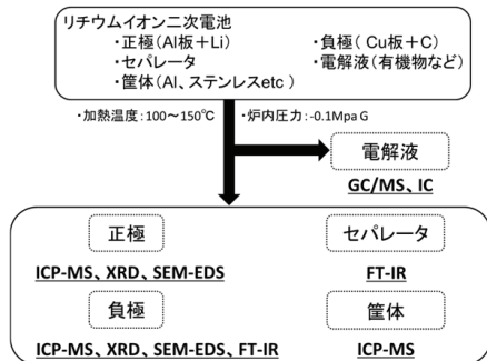
図2 ターゲット部品と分析装置
