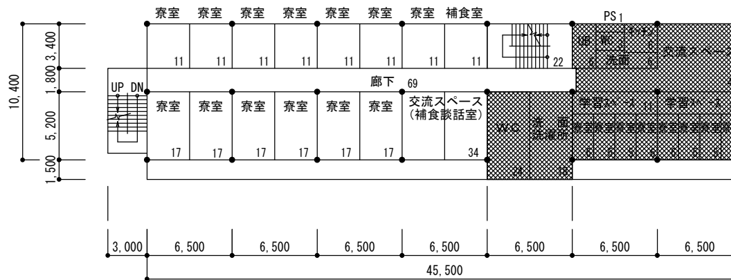
松韻寮（北寮）4階改修後平面図（491m 2 ） S=1/400
