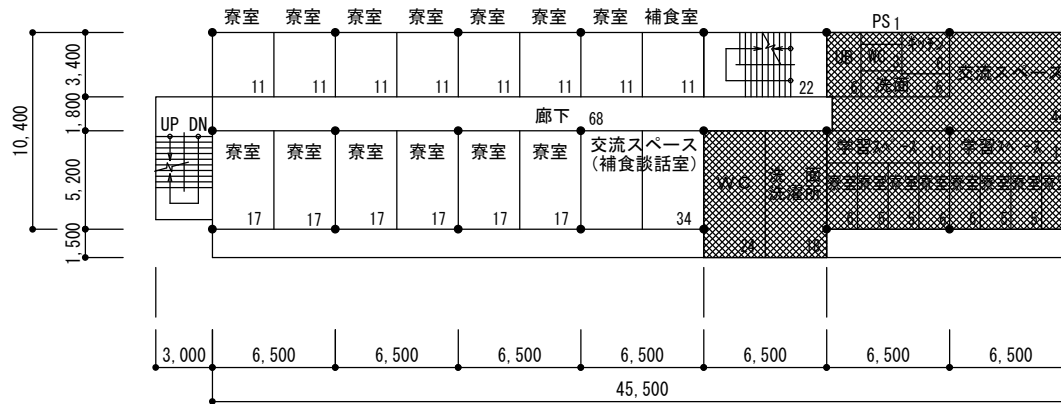
松韻寮（北寮）2階改修後平面図（490m 2 ） S=1/400
