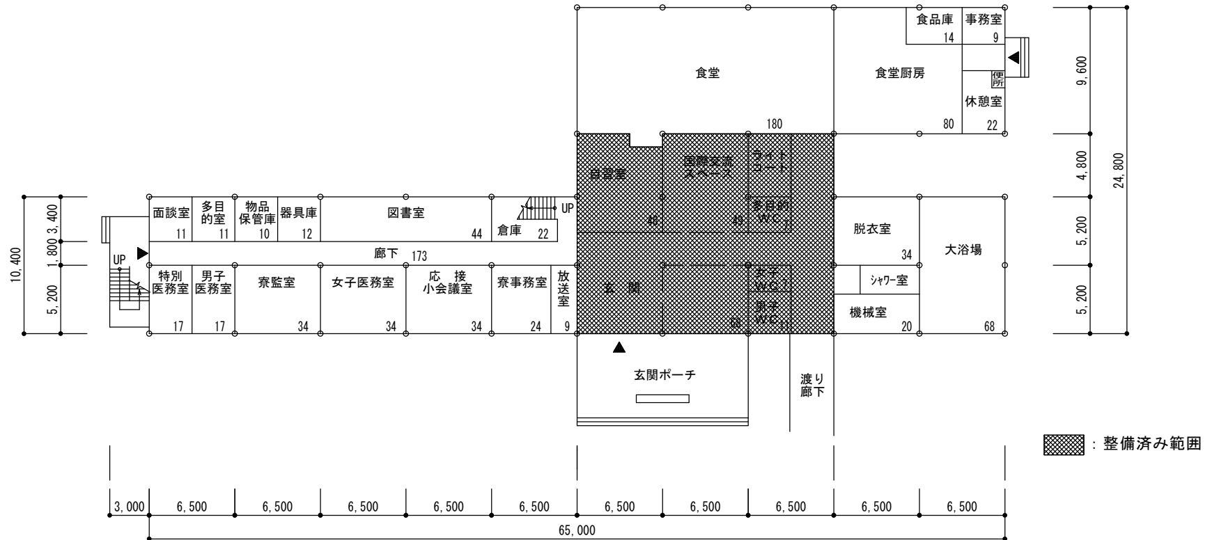
松韻寮（北寮）1階改修前平面図（1,062m 2 ）S=1/400
