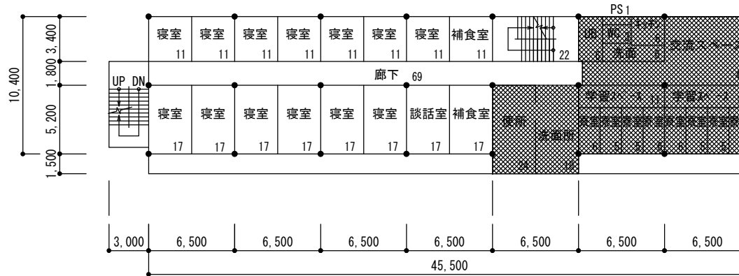
松韻寮（北寮）4階改修前平面図（491m 2 ） S=1/400
