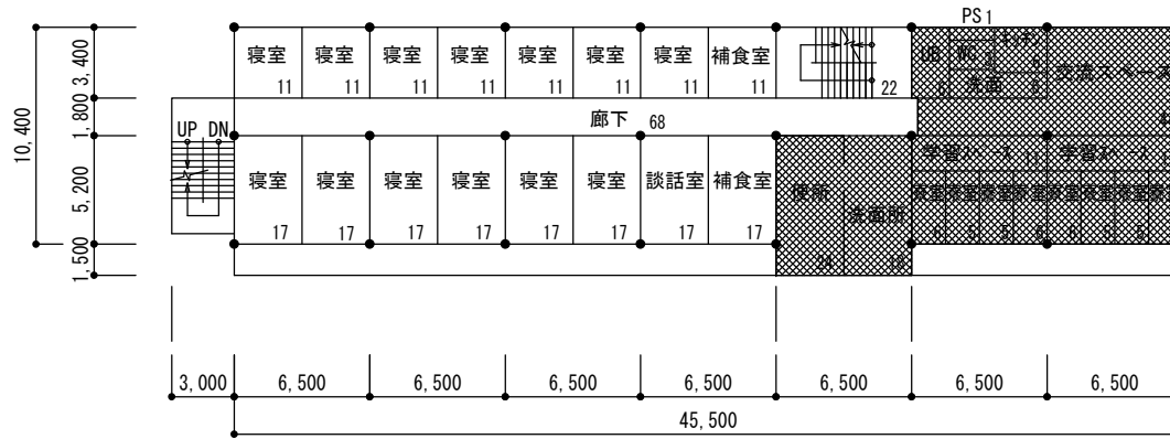
松韻寮（北寮）2階改修前平面図（490m 2 ） S=1/400
