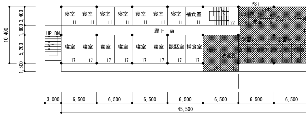
松韻寮（北寮）3階改修前平面図（491m 2 ） S=1/400
