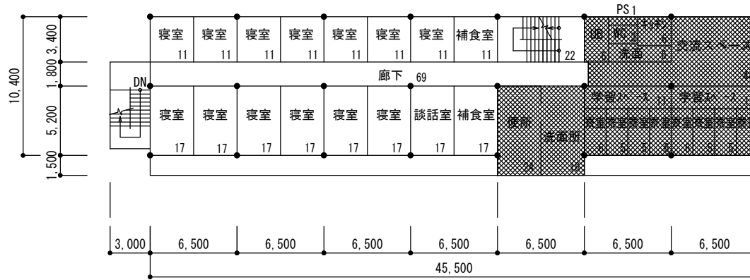
松韻寮（北寮）5階改修前平面図（491m 2 ） S=1/400
