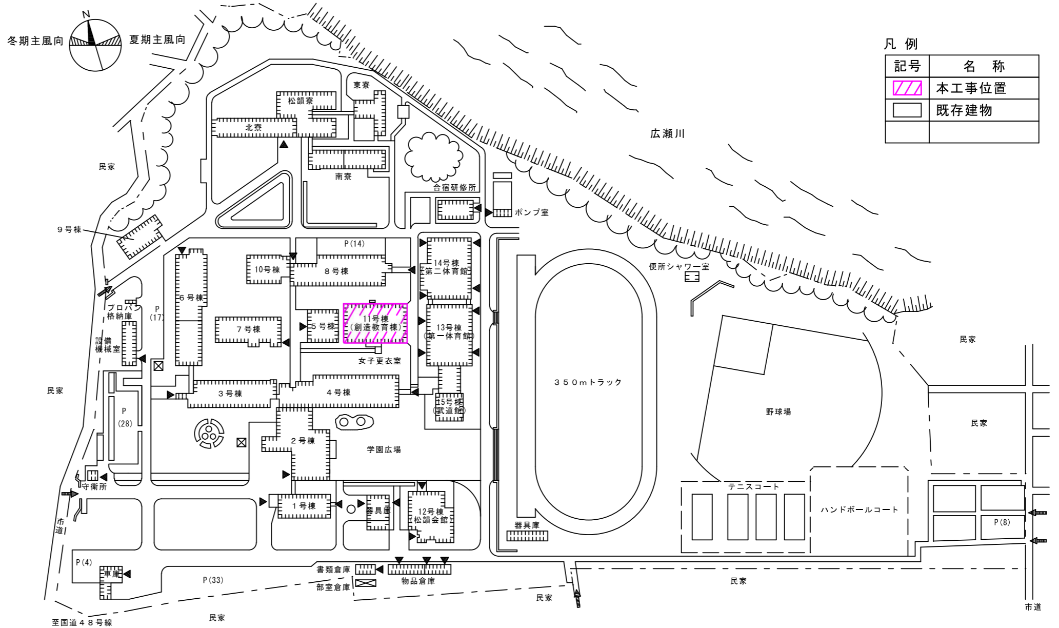
配置図 S=1/3,000
