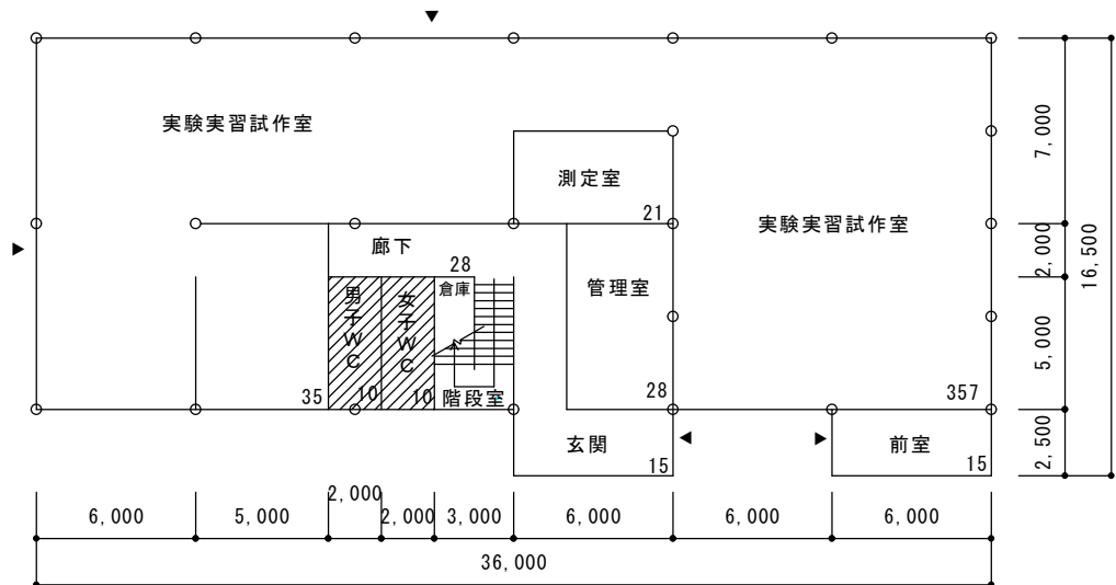
7号棟 1階改修前平面図 (534m 2 ) S=1/500
