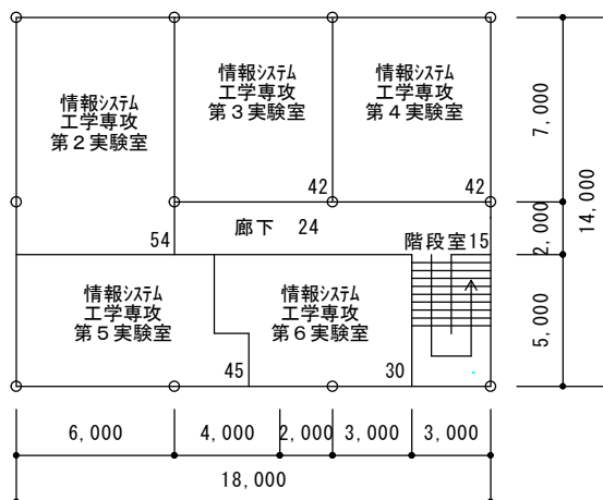
7号棟 2階改修前平面図 (252m 2 ) S=1/500
