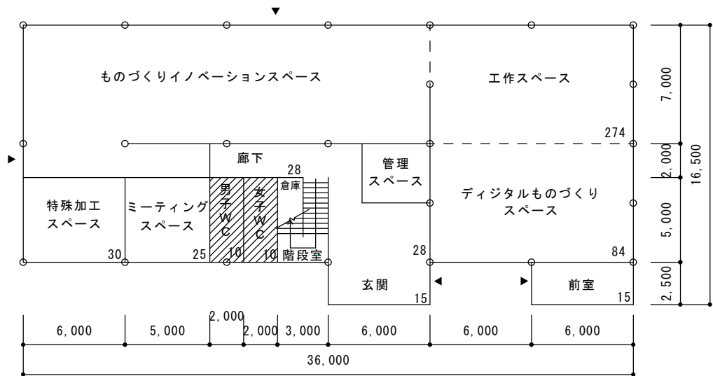
7号棟 1階改修後平面図 (534m 2 ) S=1/500
