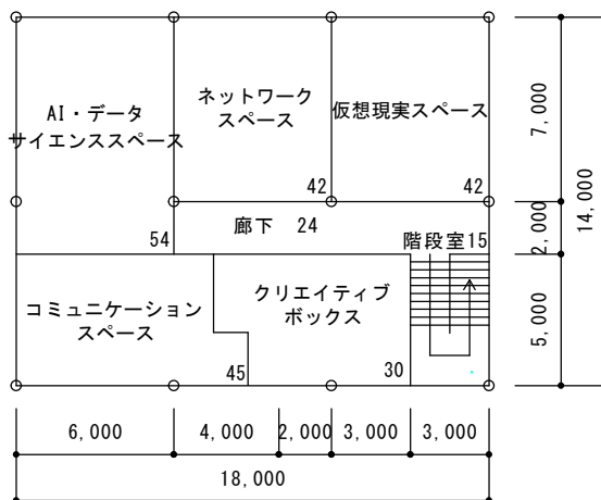
7号棟 2階改修後平面図 (252m 2 ) S=1/500
