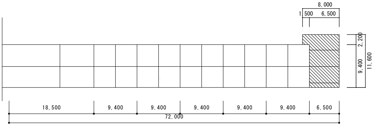
南立面图
