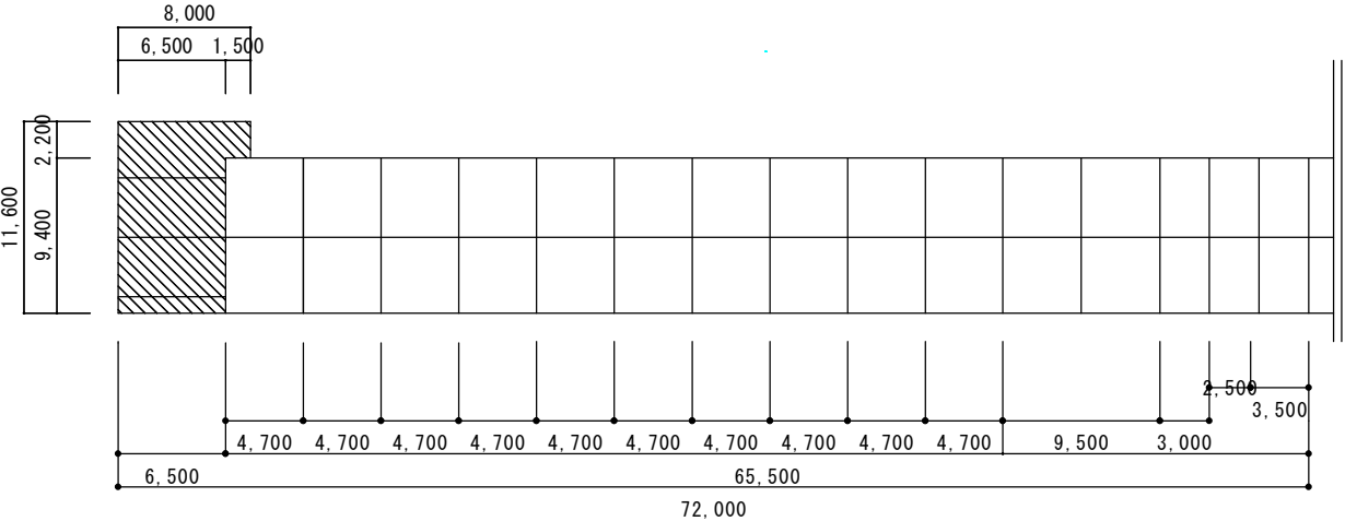
北立面图
