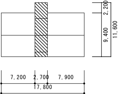
東立面图
