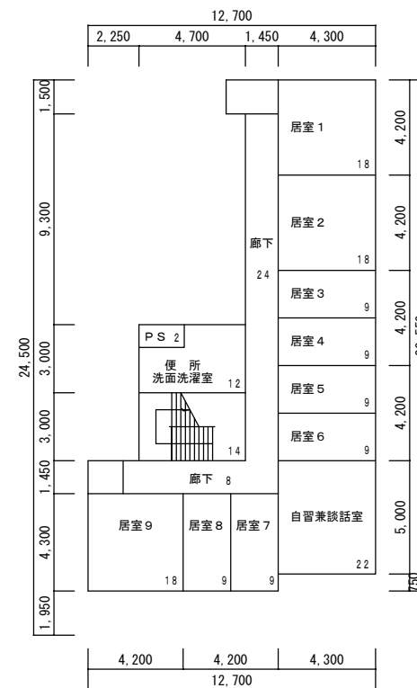
女子寮 3 階 185m 2
