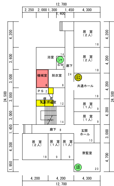
南西寮 1階 239m 2
