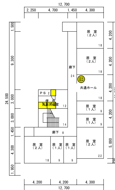
南西寮 3階 185m 2
