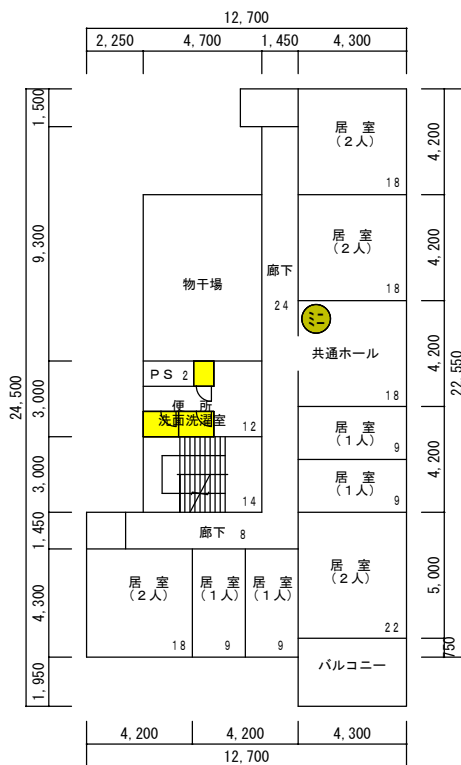
南西寮 2階 186m 2
