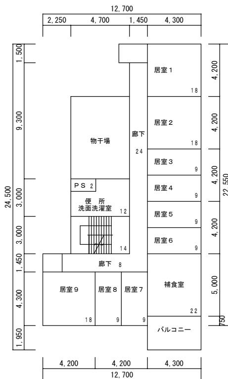
女子寮 2 階 186m 2
